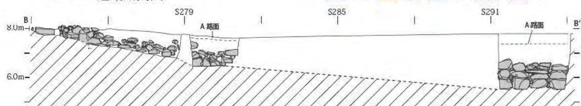
SX2900 石垣側面図
