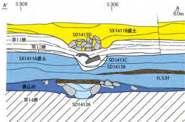
SD1413横断面(図版6A-A')
