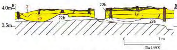
SX2968・SA2967側面図
