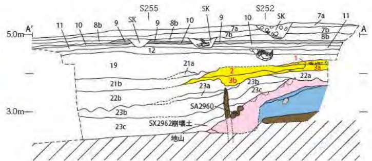
西壁断面図
