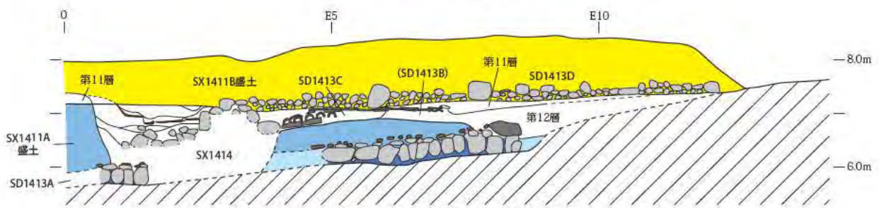
SD1413暗渠東西方向模式図
